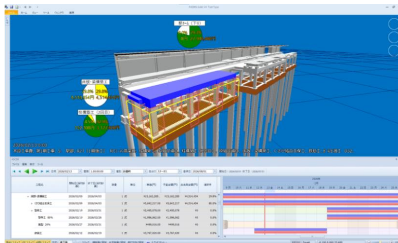
5次元施工シミュレーションシステム ※サンプル画面
